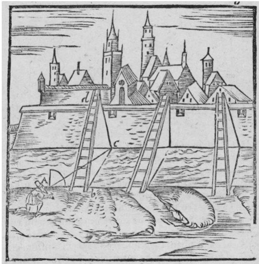
Illustration fra Thomas Finckes bog Geometriæ Rotundi fra 1583.
